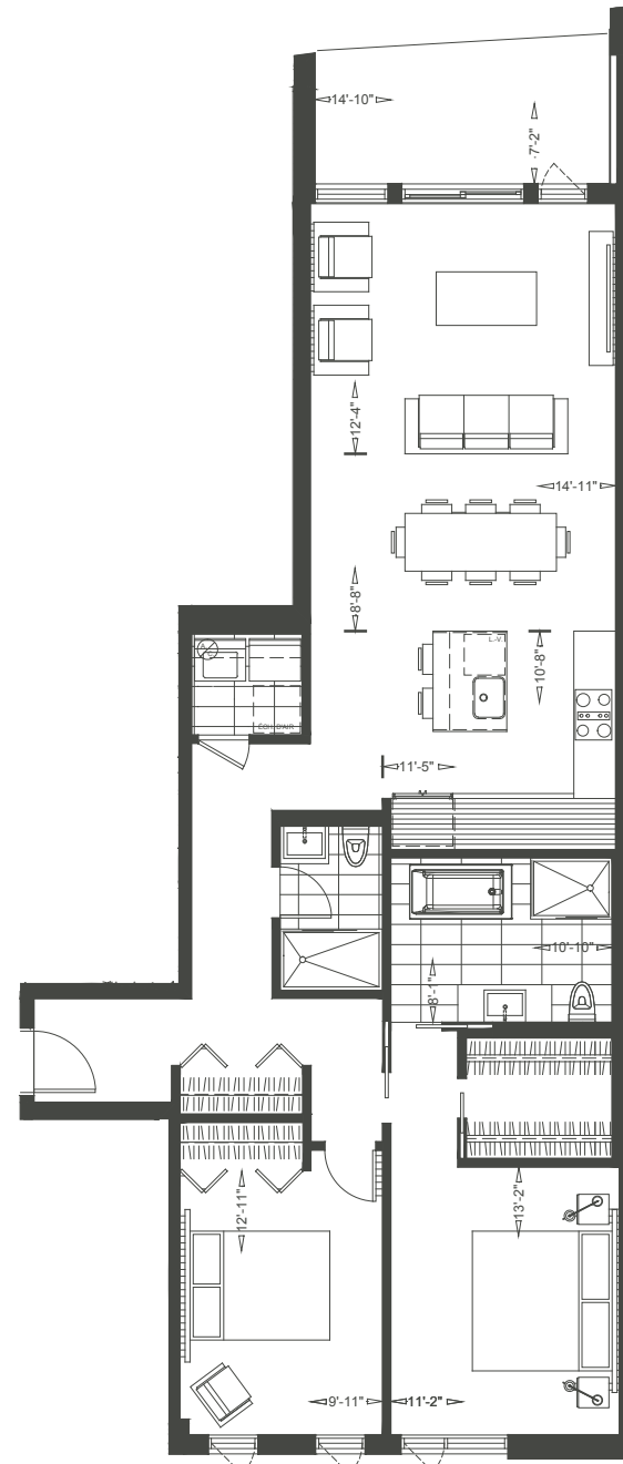
plan étage
